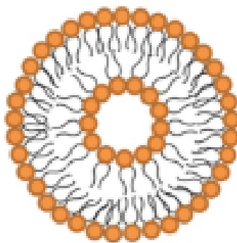
Liposomes
