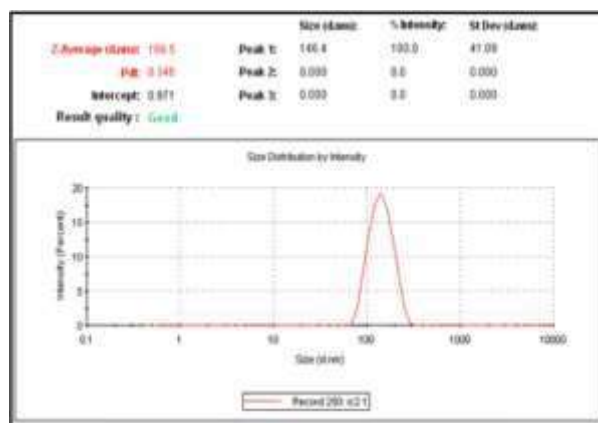
Fig 7 : .Particle size distribution of CS-NPs-8
